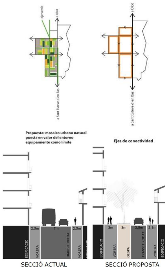
Figura 5. Planta i esquema del desdoblament de la carretera N-152 en el municipi de les Preses. Secció de la N-152 al seu pas per les Preses. Secció actual i secció proposada. Font: Magrinyà 2015
